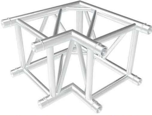
40x40 Kare Truss - 2 Yollu L Köşe
