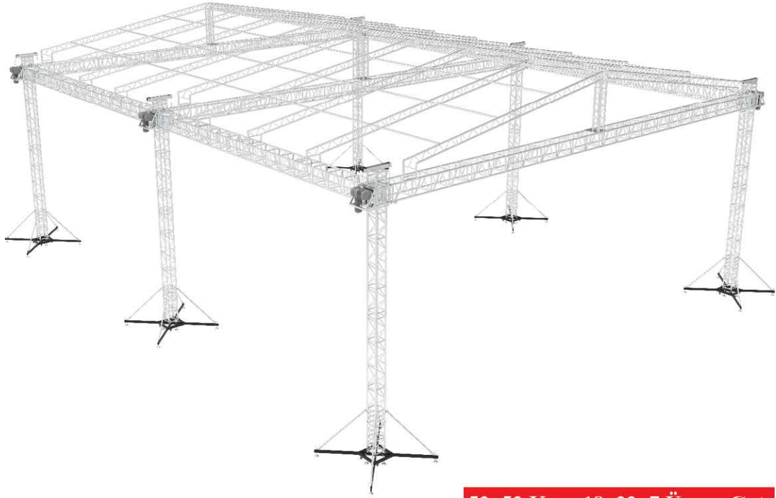
52x52 Kare 18x22x7 Üçgen Çatı
