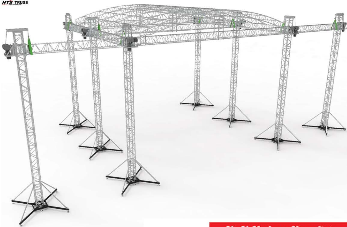
52x52 Katlanır Uzay Çatı
